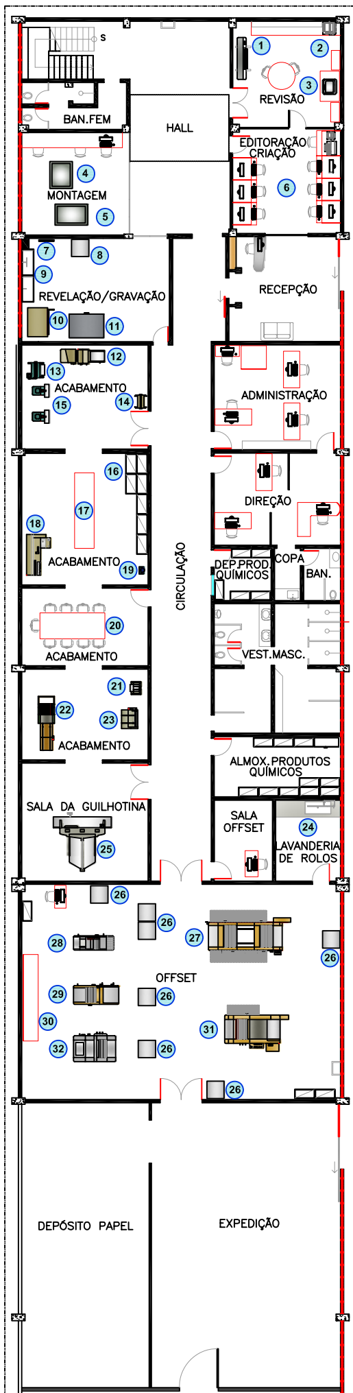
PLANTA BAIXA - LAYOUT - MÁQUINAS / EQUIPAMENTOS E OUTROS
