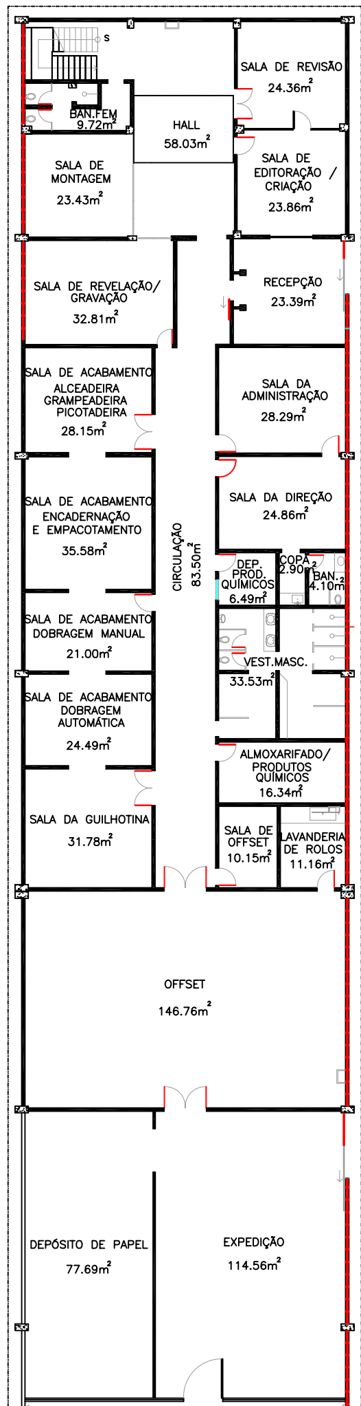
PLANTA BAIXA 1º E 2º PAVIMENTO DIVISÃO GRÁFICA DA UFRJ
