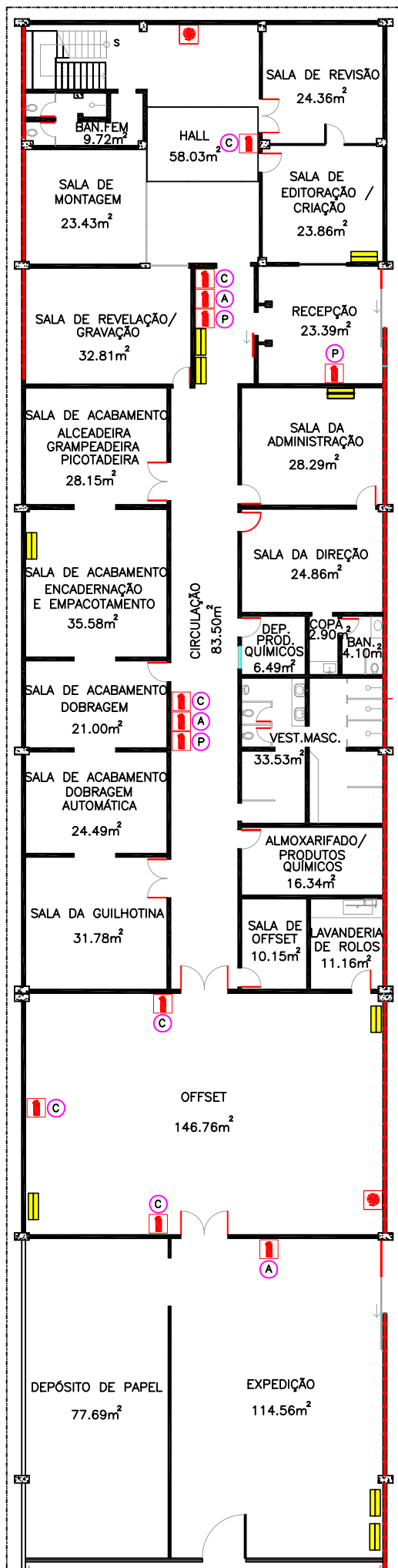
PLANTA BAIXA 1º PAVIMENTO
